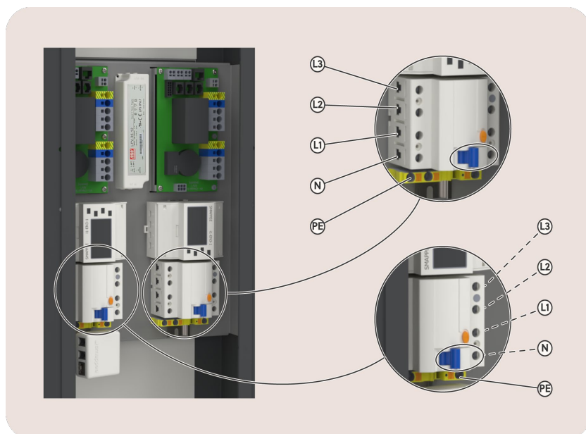
Afbeelding 12: Aanzicht op de voedingsaansluiting
