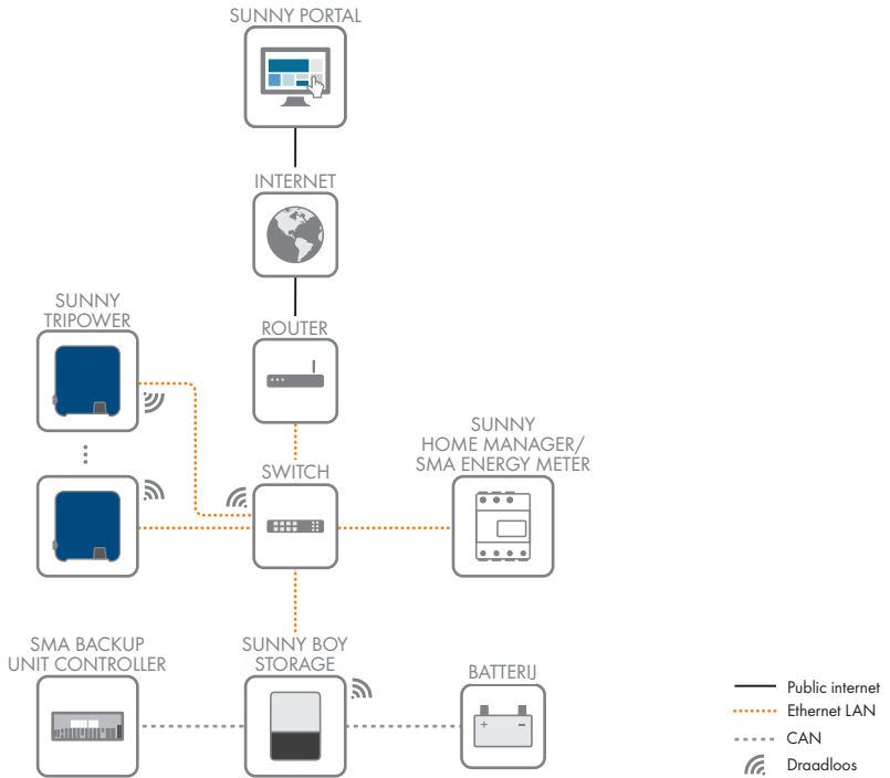
Afbeelding 4: Structuur installatiecommunicatie
