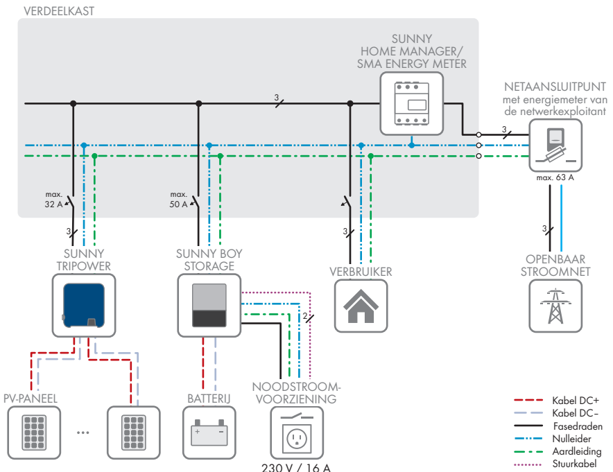
Afbeelding 3: Schakelschema (voorbeeld)
