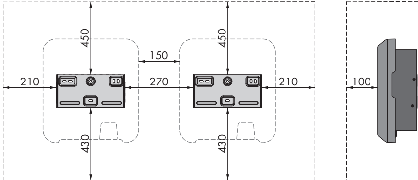
Afbeelding 7: Aanbevolen afstanden (afmetingen in mm)
