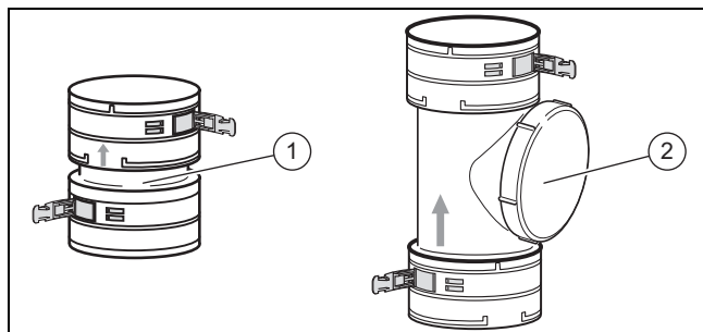
1 Verbindingselement 2 Reinigingselement
